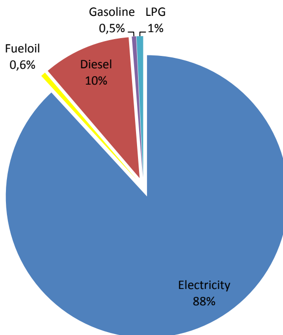
Διάγραμμα 3.27. BAU σενάριο – Εκπομπών CO 2 τελικής χρήσης ανά ενεργειακό φορέα το 2020
