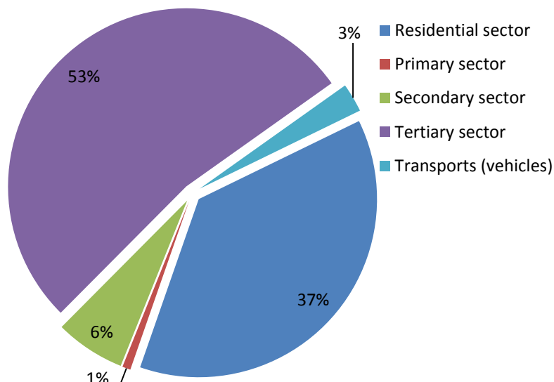
Διάγραμμα 3.13. Κατανομή συνολικών εκπομπών CO 2 από τελική χρήση στους διάφορους τομείς
